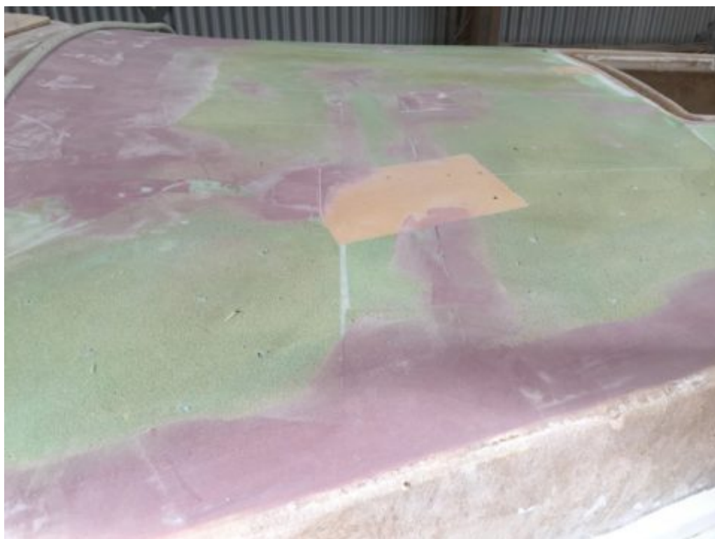
Étape intermédiaire : dégommage du sandwich dans le cockpit et remplacement par de la mousse
